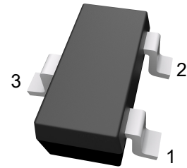
1.GND 2.VOUT 3.VIN
